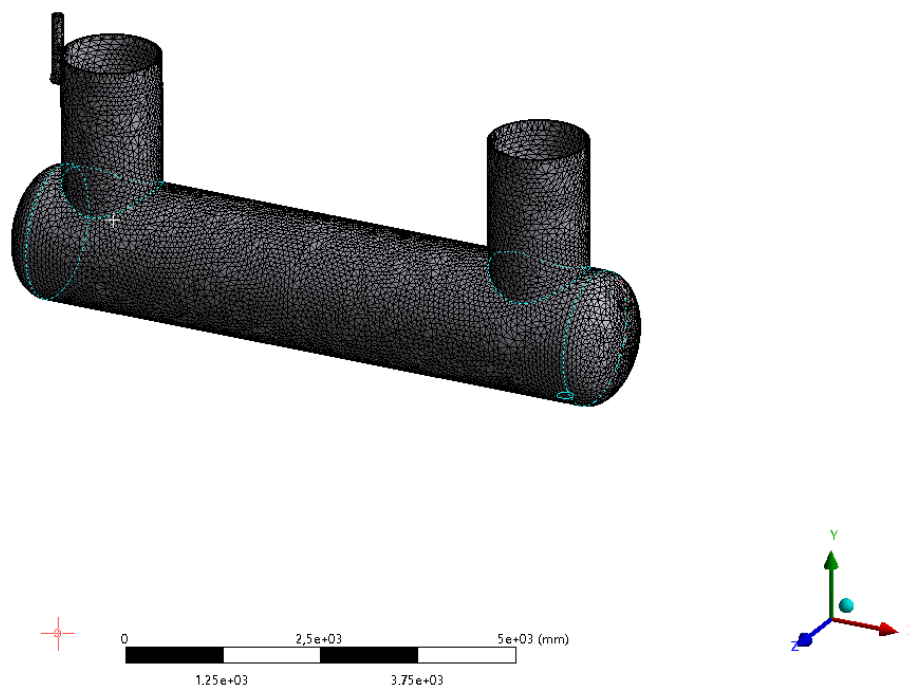
Рис. 3. Расчетная аппроксимированная модель Определение собственных частот колебаний изделия:
