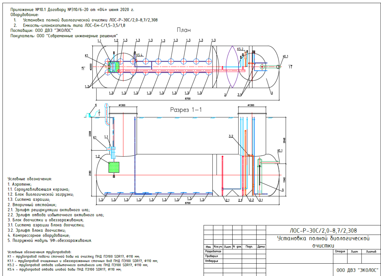
Рис. 1 Общий вид.
